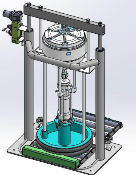
55加仑气动打胶升降机3D建模图
