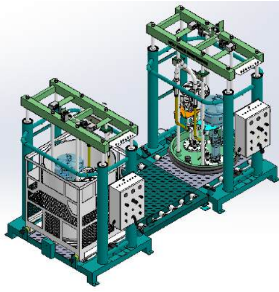
1000L气动打胶升降机3D建模图
