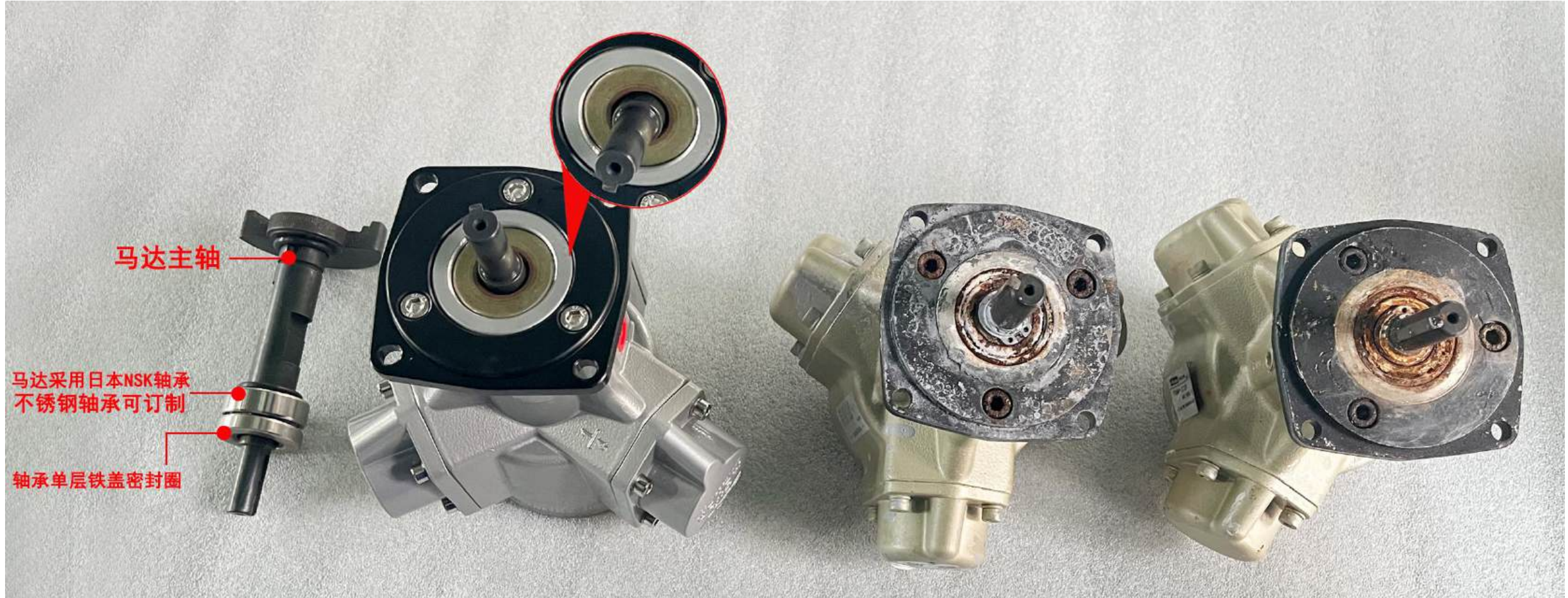
德斯威日标型活塞式气动马达内部轴承结构图
