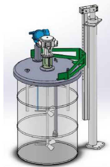
走珠系统55加仑气动升降搅拌机3D建模图
